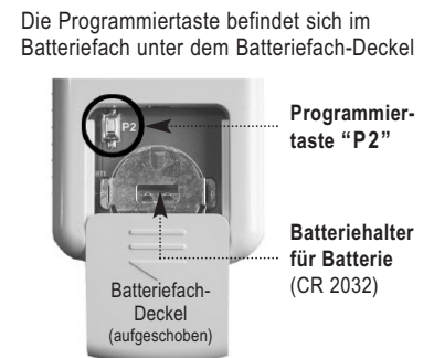
(Abb. 3) Rückseite:
